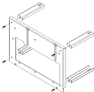
Figura 31 – Montagem mesa auxiliar
