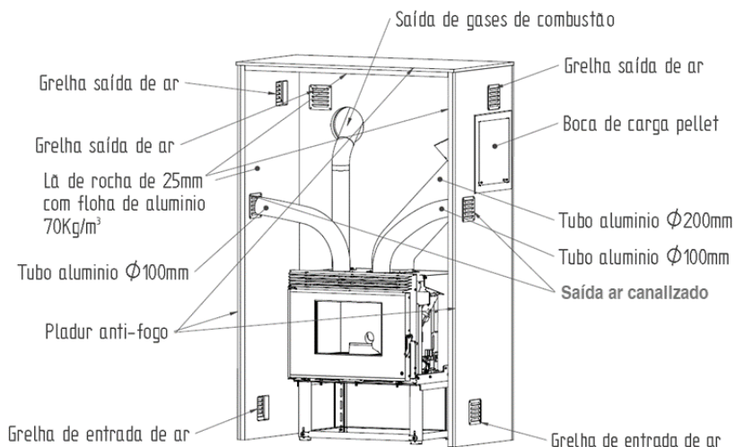
Figura 22 – Instalação inserível a pellets
