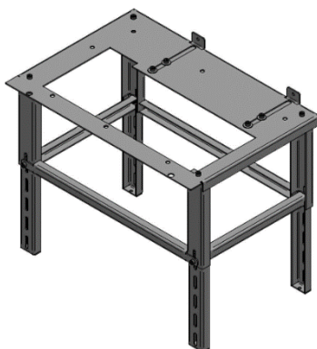
Figura 30 – Instalação de mesa auxiliar
