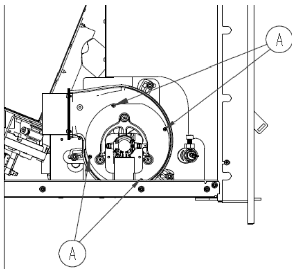
Figura 50 – Verificação dos parafusos PH2
