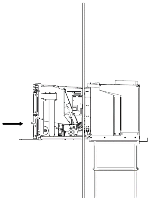
Figura 12 – Instalação inserível
