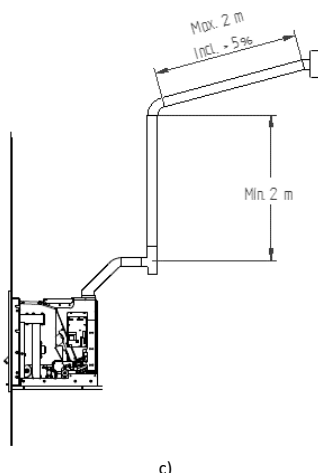
Figura 2 – Exemplos de instalações tipo
