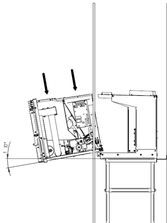
Figura 10 – Instalação inserível
