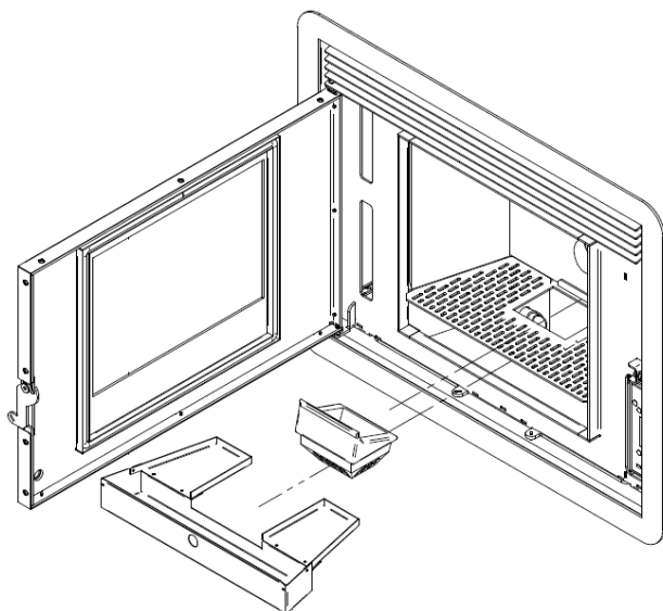
Figura 44 – Remoção dos componentes cesto de queima, grelha e cesto de cinzas
